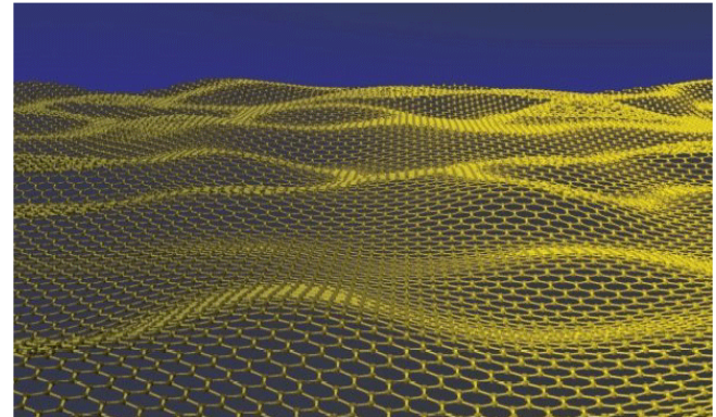
Physique théorique (LPTMC) Ondulation transversales d'une monocouche de graphène
