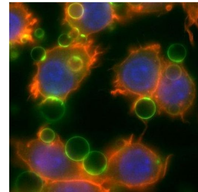
Biophysique (LJP - LPTMC - PCC) Contrôle la déformation dans des émulsions biomimétiques
