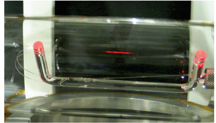
Miroir de Bragg avec qq milliers atomes; Julien Laurat (LKB)
